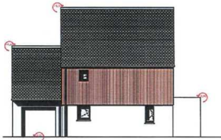
façade nord-est
